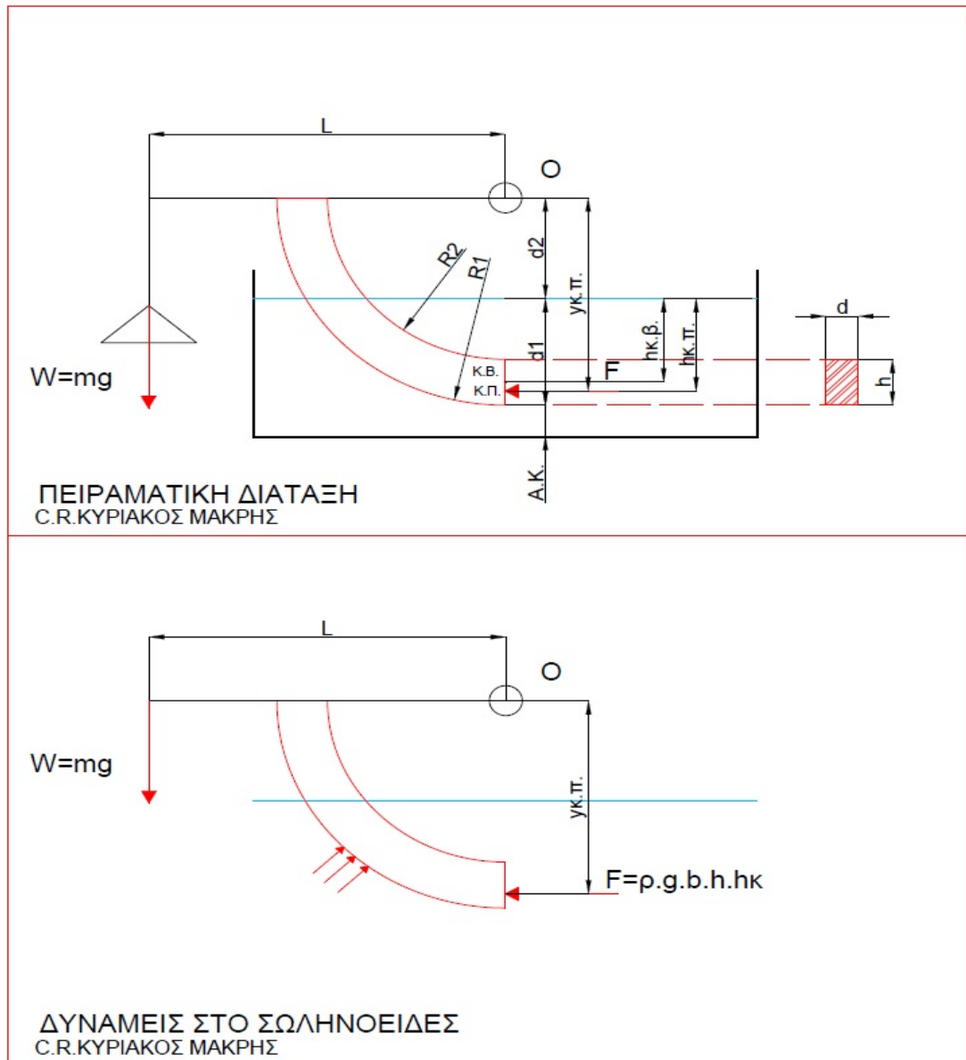
Σχήμα 1. Παρουσίαση Πειραματικής Διάταξης
