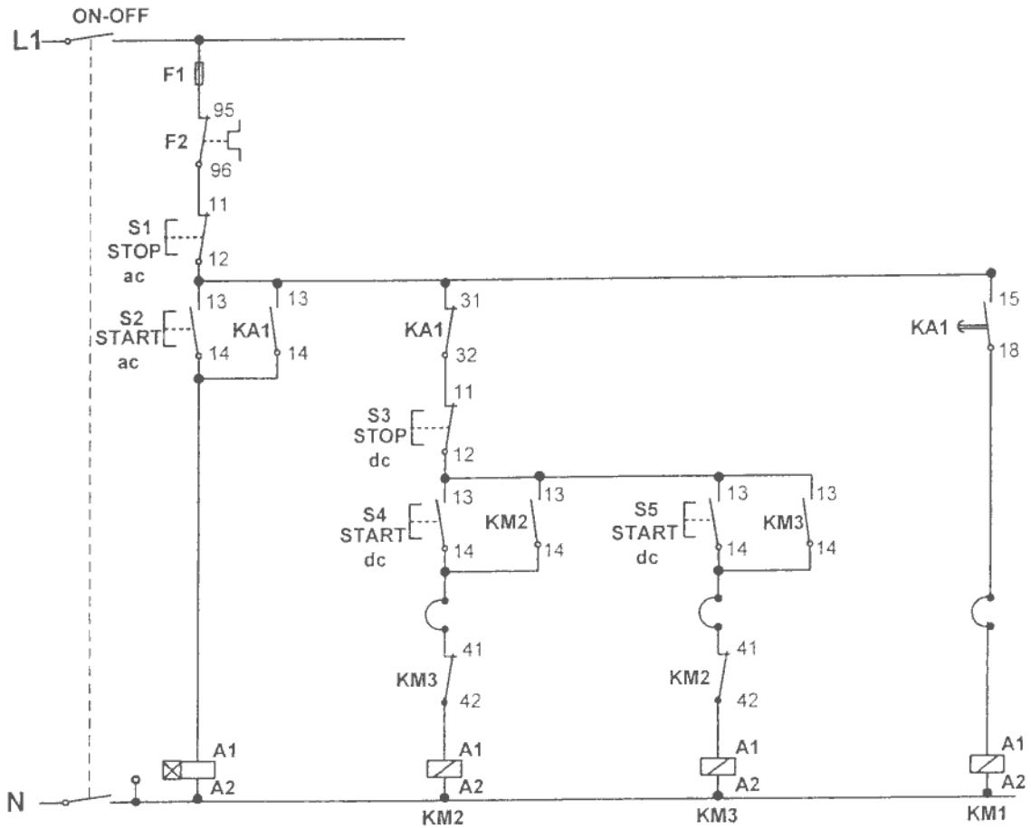
ΚΥΚΛΩΜΑ ΕΛΕΓΧΟΥ
