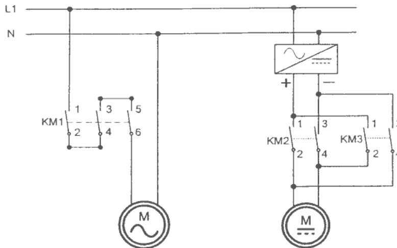
ΚΥΚΛΩΜΑ ΙΣΧΥΟΣ
