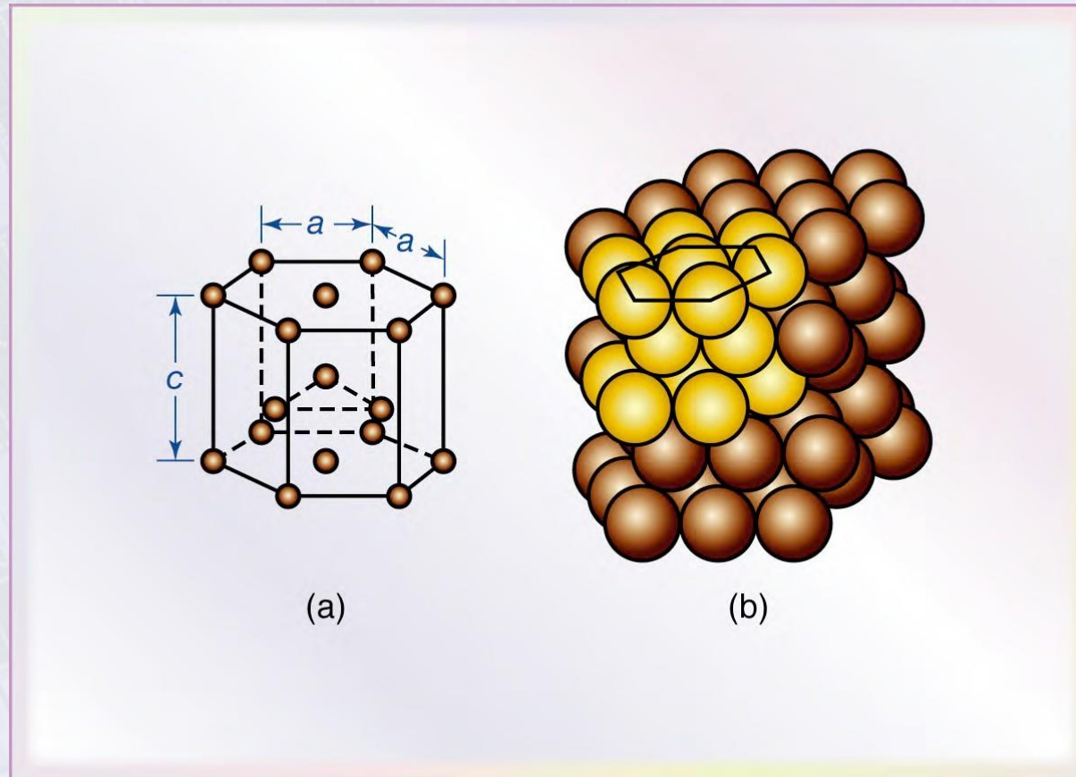
Figure: Η κρυσταλλική δομή hcp (εξαγωνική διάταξη μέγιστης πυκνότητας): (α) μοναδιαία κυψελίδα και (β) μονοκρύσταλλος με πολλές μοναδιαίες κυψελίδες.
