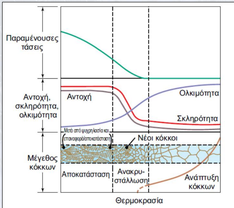
Figure: Επιδράσεις της ανάκτησης, ανακρυστάλλωσης και ανάπτυξης κόκκων στις μηχανικές ιδιότητες και στο σχήμα και μέγεθος των κόκκων· παρατηρήστε τον σχηματισμό νέων, μικρών κόκκων κατά τη διάρκεια της ανακρυστάλλωσης. Πηγή: G. Sachs.
