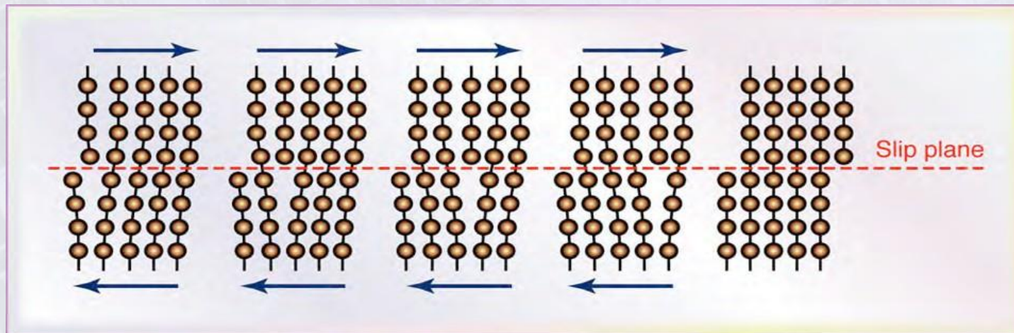
Figure: Κίνηση μιας διαταραχής ακμής κατά μήκος του κρυσταλλικού πλέγματος υπό διατμητική τάση. Η ύπαρξη διαταραχών εξηγεί γιατί η πραγματική αντοχή των μετάλλων είναι μικρότερη από τη θεωρητικά προβλεπόμενη.
