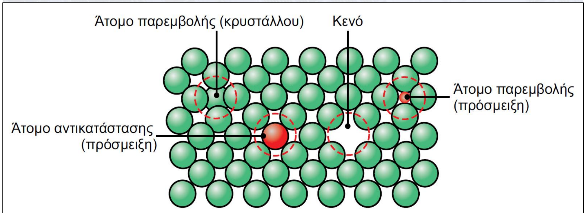
Figure: Σχηματική αναπαράσταση των διάφορων τύπων ατελειών σε πλέγμα μονοκρυστάλλου.
