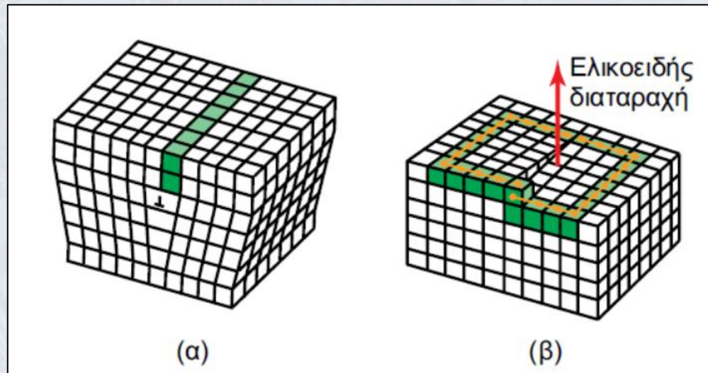
Figure: Τύποι διαταραχών σε μονοκρυστάλλο: (α) διαταραχή ακμής και (β) ελικοειδής διαταραχή.
