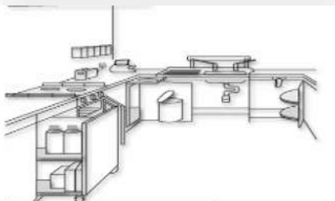
Εικόνες 165 & 166. Κουζίνα για χρήση αμαξιδίου (αριστερά) και υποδοχές ερμαρίων (δεξιά) (Υ.Π.ΕΝ., 2020)
