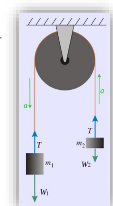
Μηχανή Atwood
